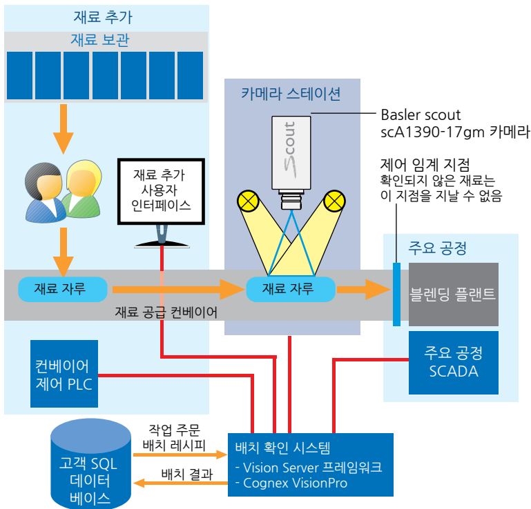
Tip Top의 새로운 아이스크림 생산 공정.
